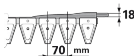
Klingenteilung beim Untermesser
